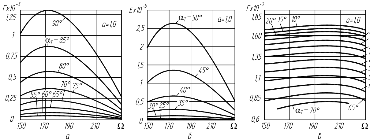
Рис. 5. Діаграми зміни точності наближення: а, б – теоретичні значення, відповідно до умов найкращого наближення за Чебишевим; в – фактичні значення, отримані числовим способом
